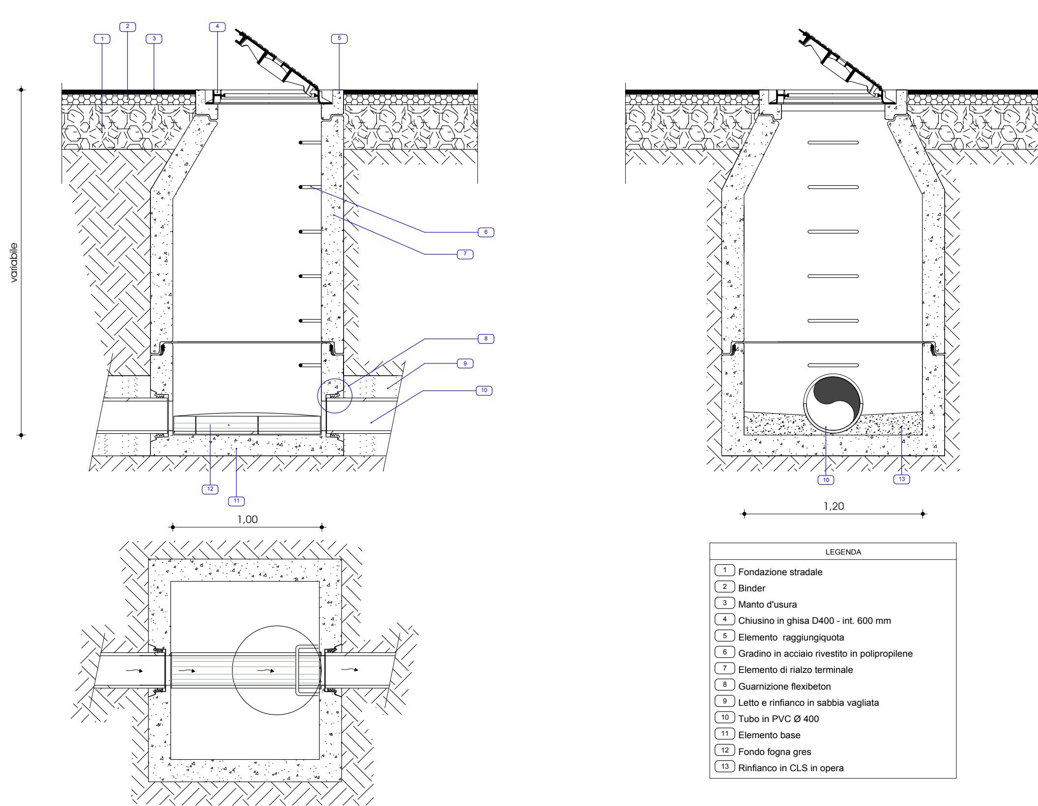
POZZETTO STRADALE DI DISPERSIONE 100X120 CON CHIUSINO IN GHISA SFERODALE D. 400
