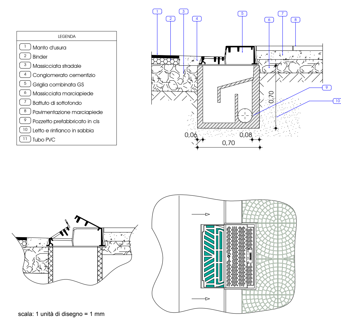
ALLACCIAMENTO FOGNARIO ACQUE MISTE AL COLLETORE MONOLITICO DI VIA LOVATO
