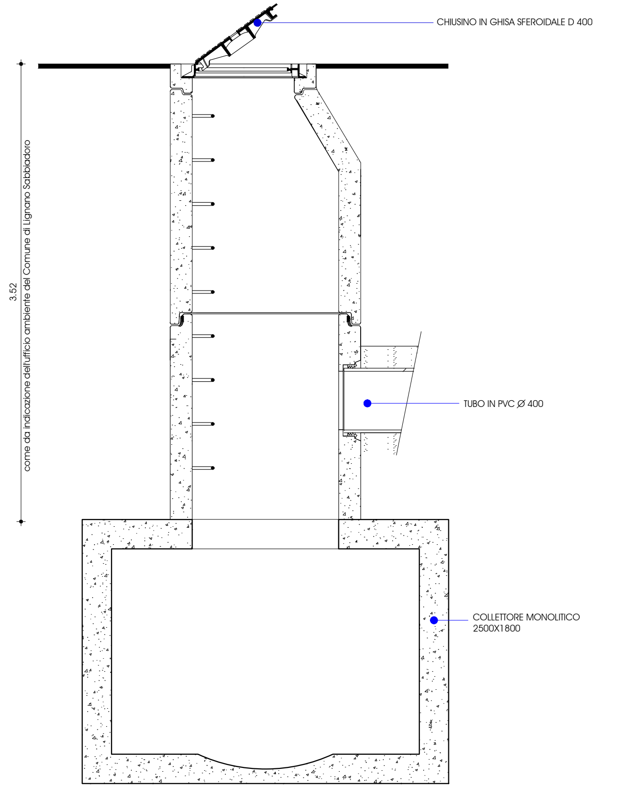
ALLACCIAMENTO FOGNARIO ACQUE MISTE AL COLLETORE MONOLITICO DI VIA LOVATO
