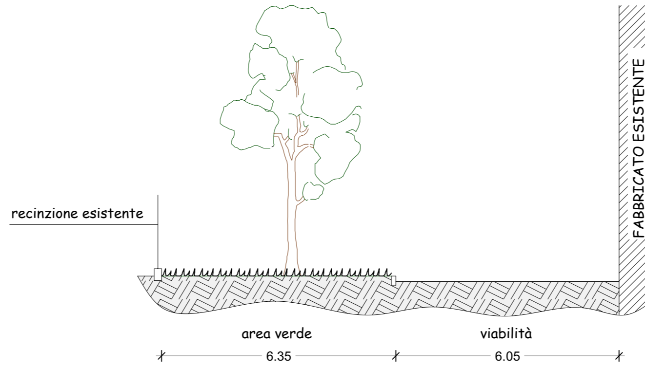
Sezione esistente sc. 1:100
