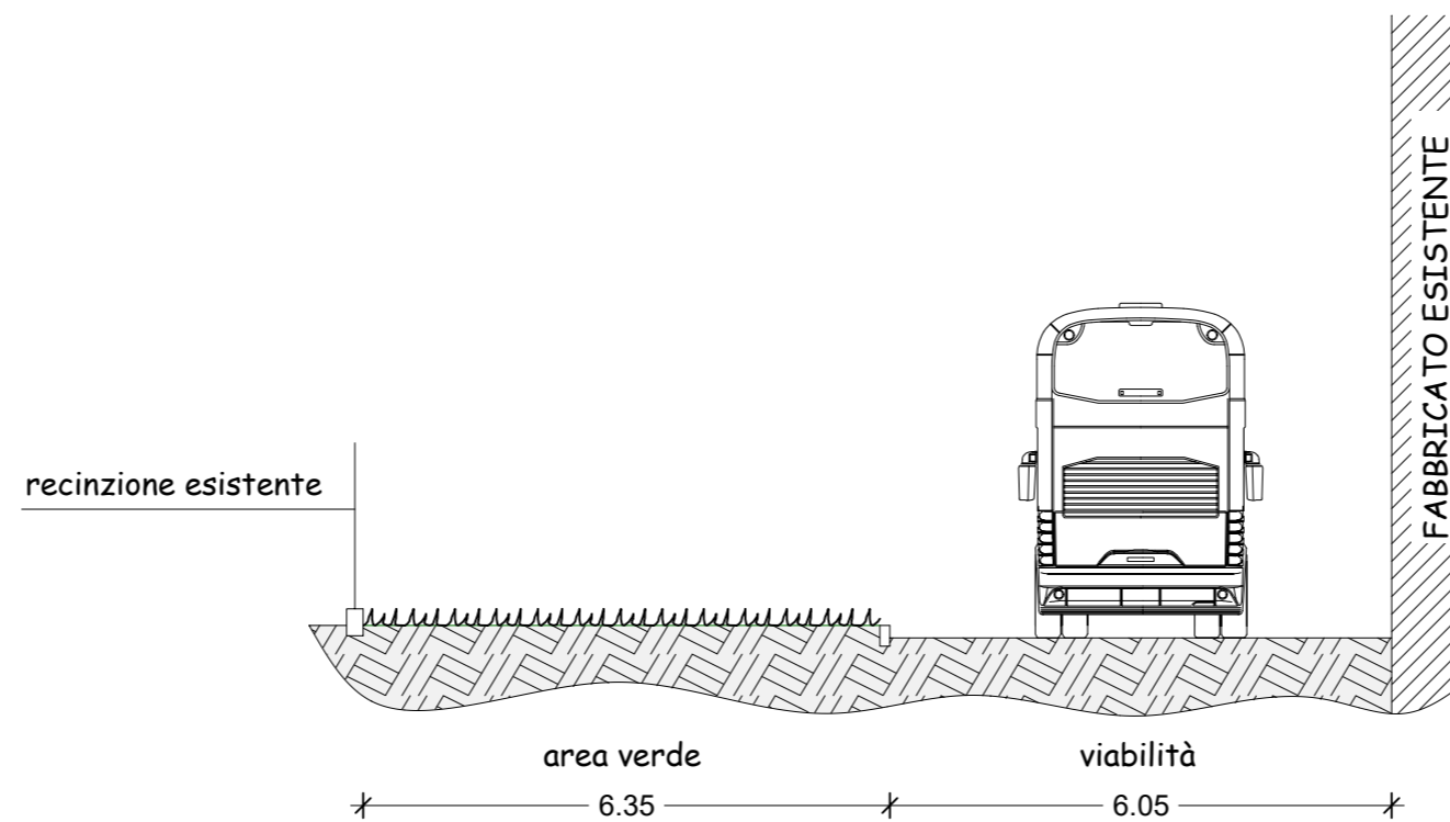
Sezione progetto sc. 1:100
