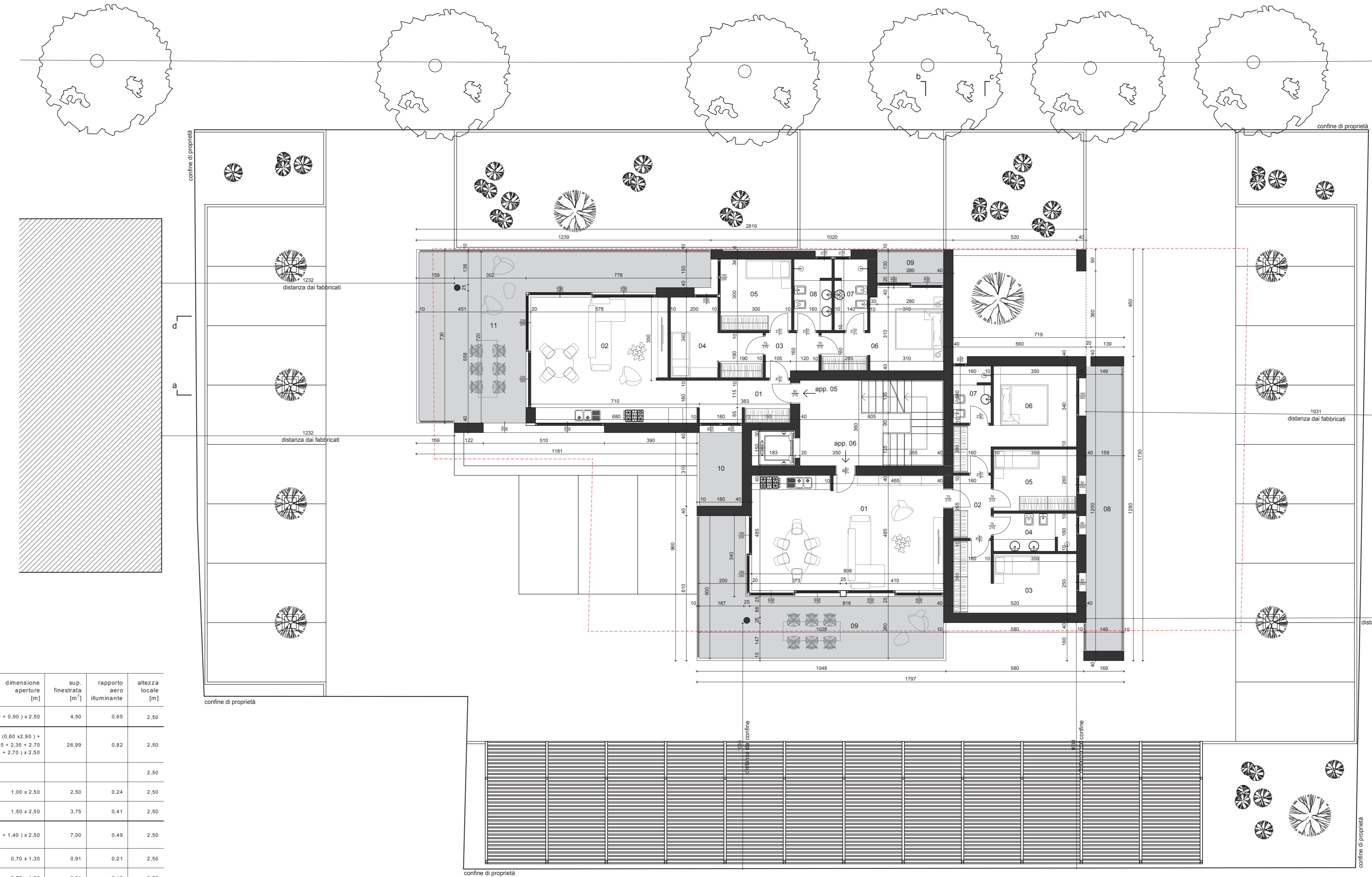
app. 06 - piano terzo
